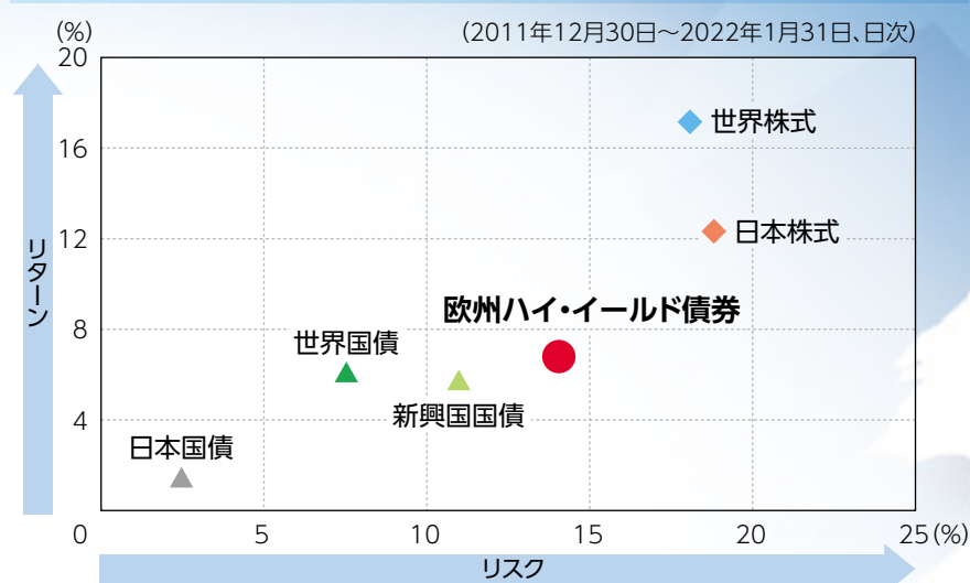
各資産のリスク・リターン分布
